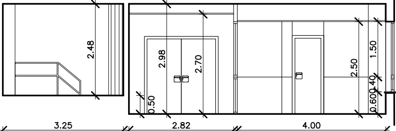
SECCION C-C' E:1/100
