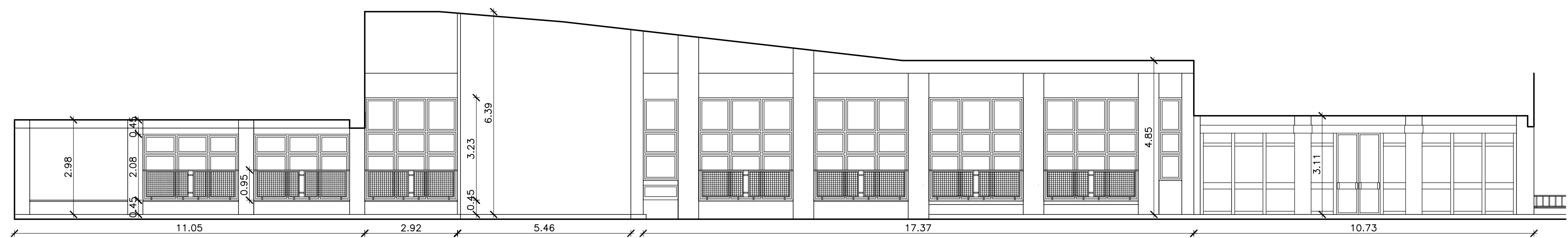
SECCION B-B' E:1/100
